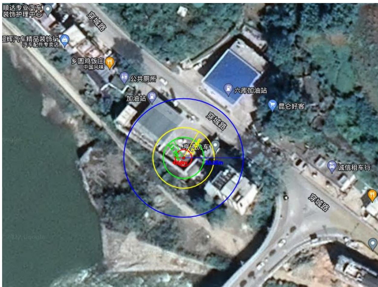
汽油罐蒸气云爆炸模拟图
